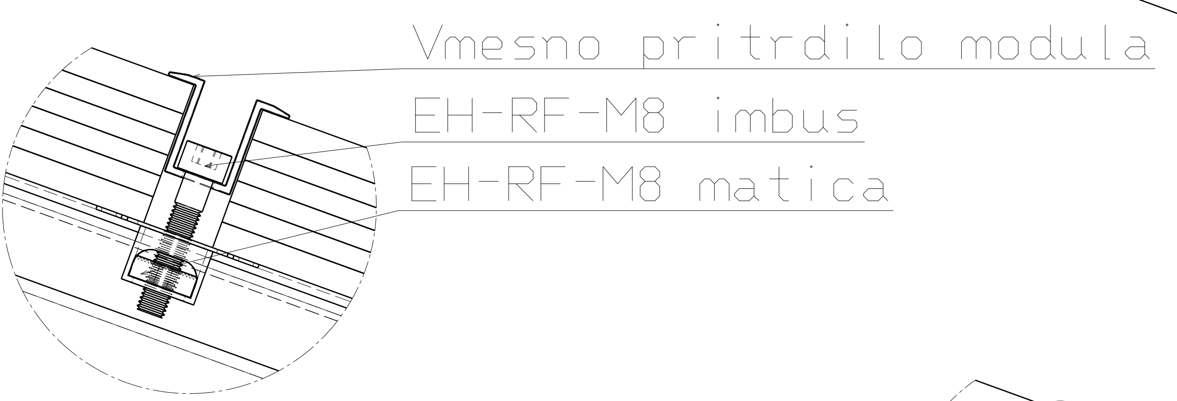
Detajl: A Scale 1:4
